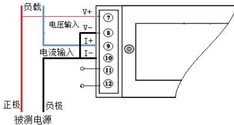
图 5.2、4223 产品电压电流端子输入时产品接线参考图
