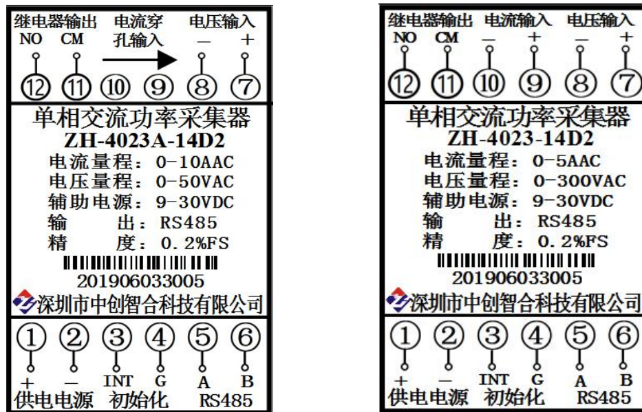
图 5.1、产品接线参考图（左图为电流穿孔输入，右图为电流 9、10 接线端子输入）
