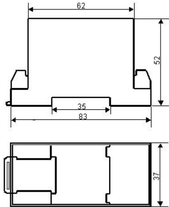
图 4.2、产品尺寸图
