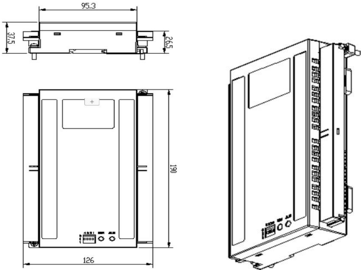
图二、外形与安装尺寸(单位: mm 安装方式: 螺钉固定)
