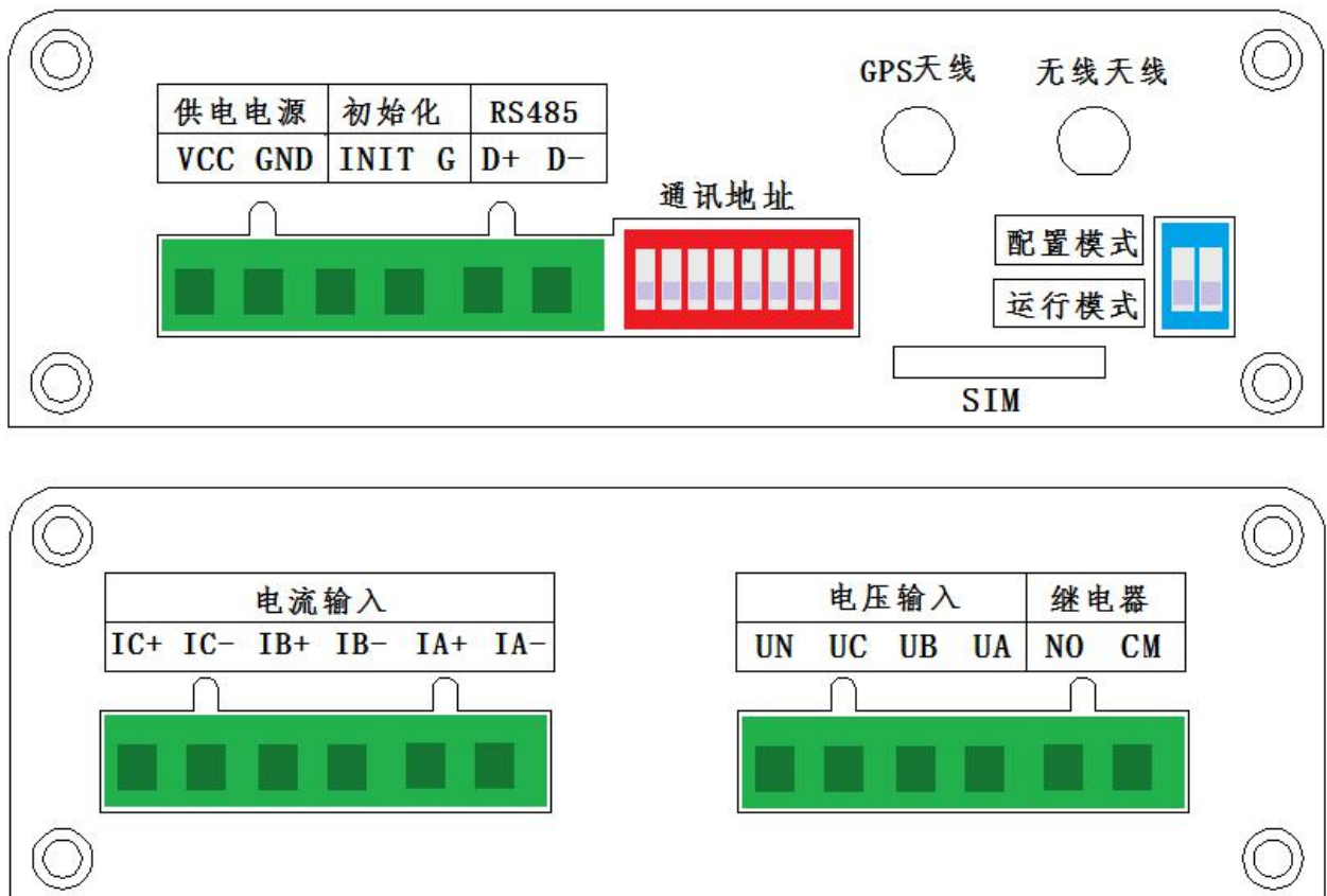
图 4.2、引脚定义图
