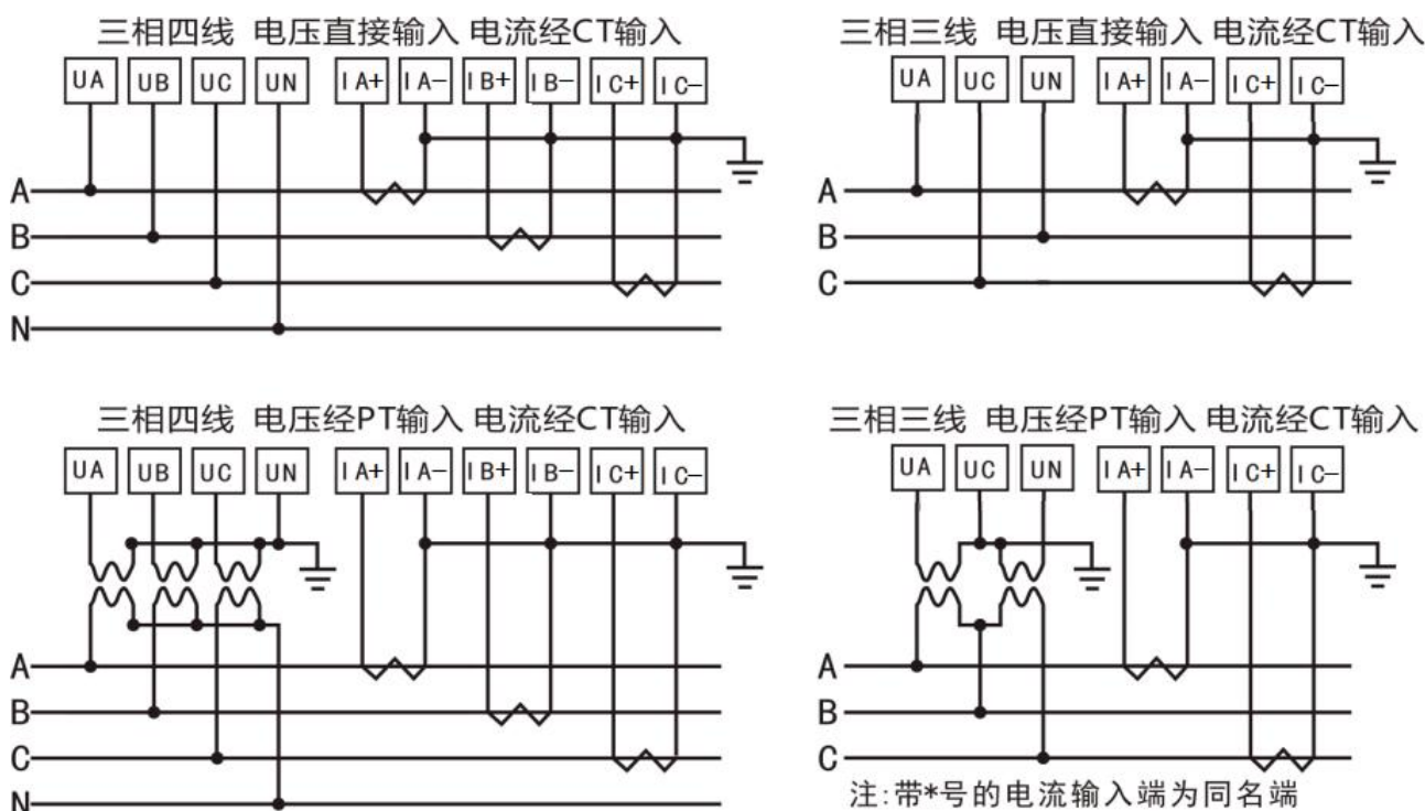
图 5.2、接线示例图
